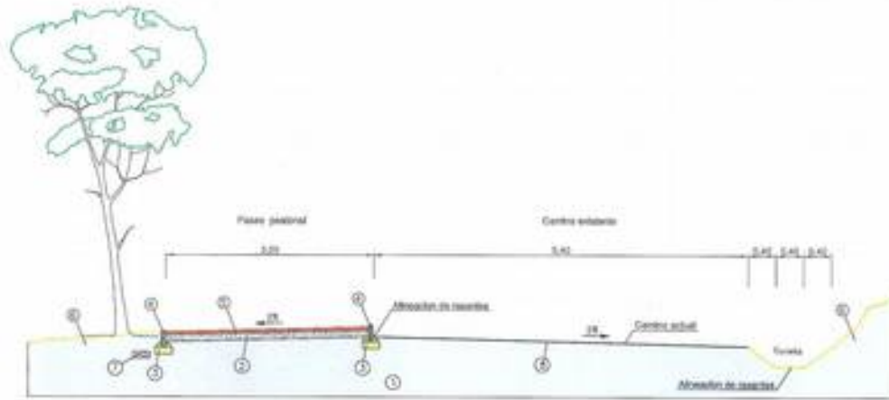
SECCION TIPO
